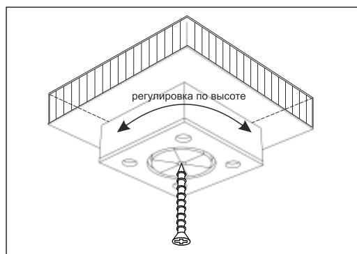
Монтаж ножки
